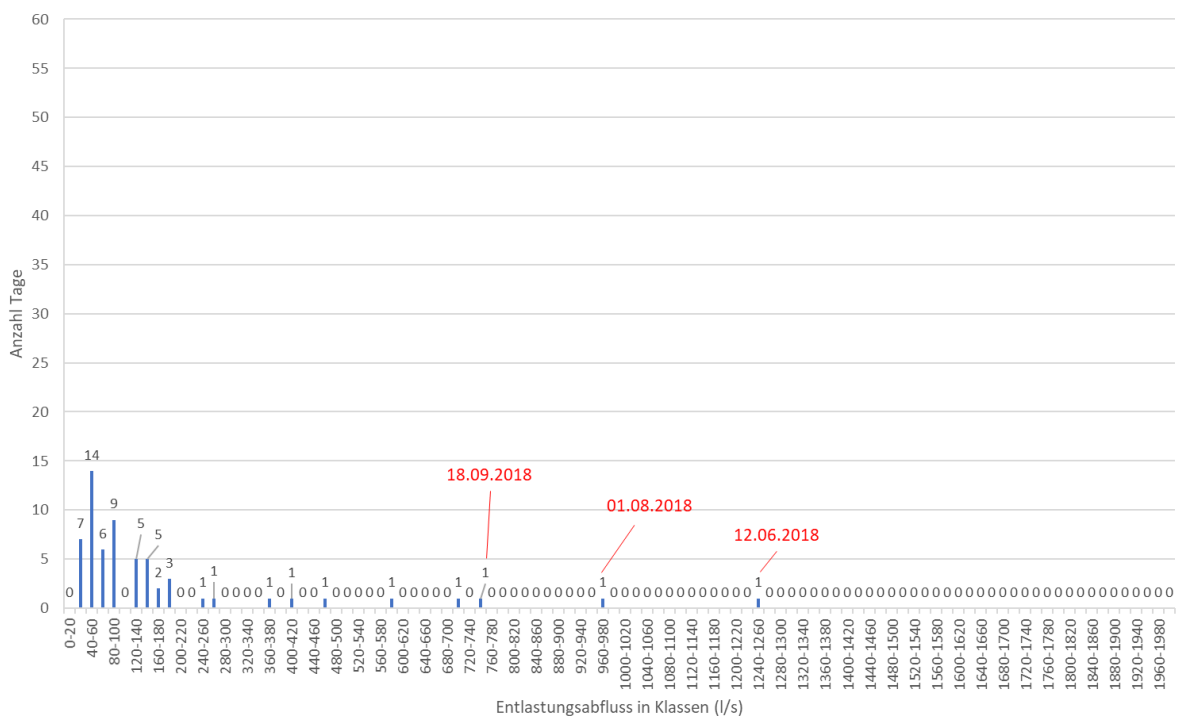
Häufigkeitsverteilung Maximaler Entlastungsabfluss (Tageswerte) RÜB Salzstetten 2018
